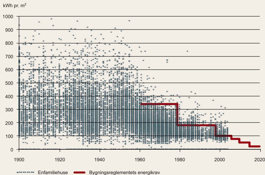
Figur 9. Energiforbrug i enfamiliehuse til opvarmning, køling, ventilation og varmt vand efter opførelsesår sammenholdt med bygningsreglementets krav
